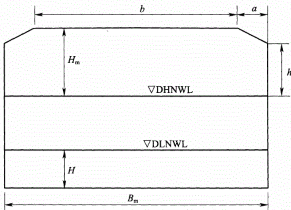
图 5.2.2 通航净空示意图
