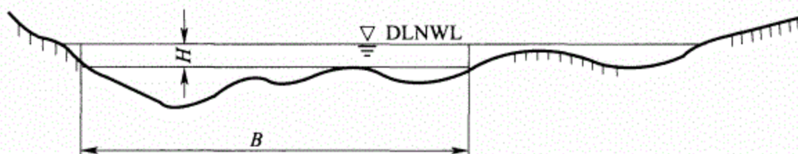
图 3.0.2 天然和渠化河流航道横断面图
