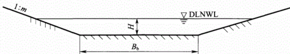
图 3.0.3 限制性航道横断面图
